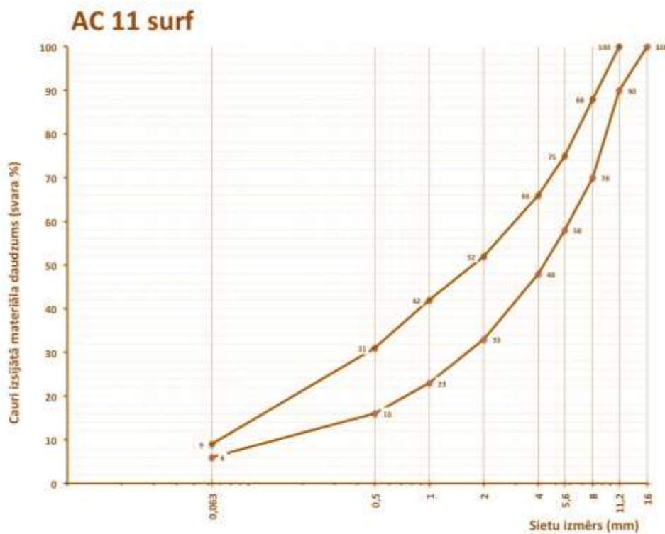
6.2-25 tabula. Prasības karstā asfalta AC 11 surf granulometriskajam sastāvam
