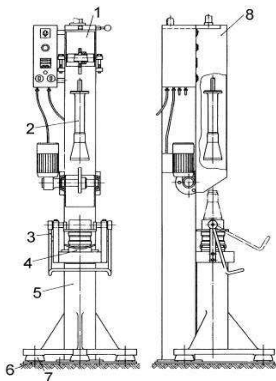
12.8-1 attēls. Trieciena blīvētāja shematisks attēls
