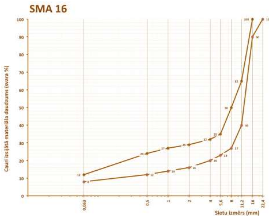
6.2-62 tabula. Prasības šķembu mastikas asfalta SMA 16 granulometriskajam sastāvam
