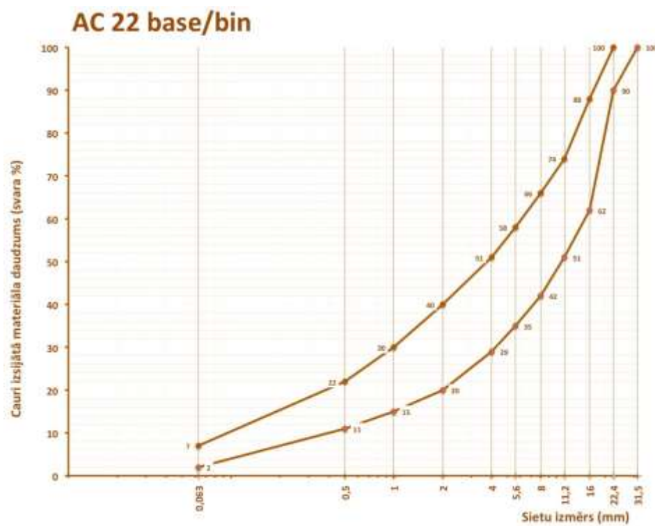
6.2-46 tabula. Prasības karstā asfalta AC 22 base/bin granulometriskajam sastāvam
