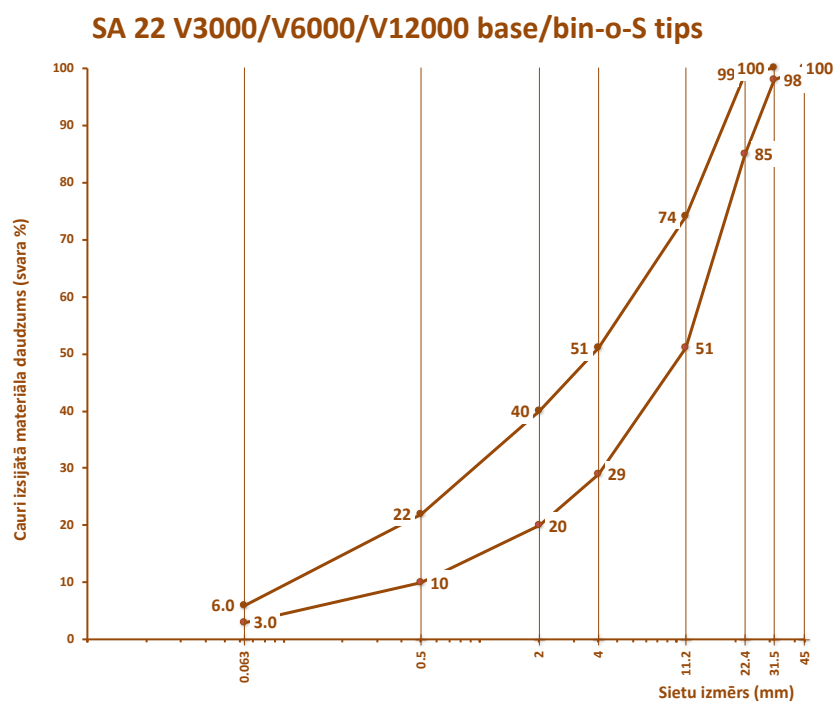
6.3-25 tabula. Prasības mīkstā asfalta SA 22 V3000/V6000/V12000 base/bin-o-S tips maisījuma granulometriskajam sastāvam
