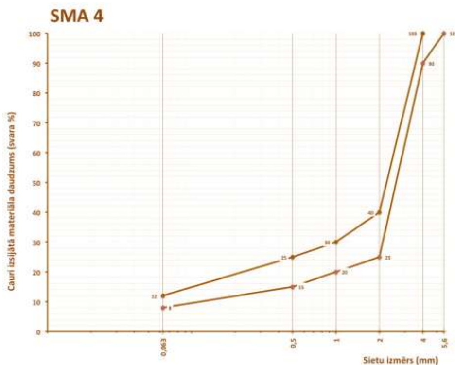
6.2-53 tabula. Prasības šķembu mastikas asfalta SMA 4 granulometriskajam sastāvam
