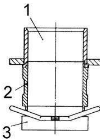
12.8-2 attēls. Trieciena blīvētāja tipiska blīvēšanas veidne
