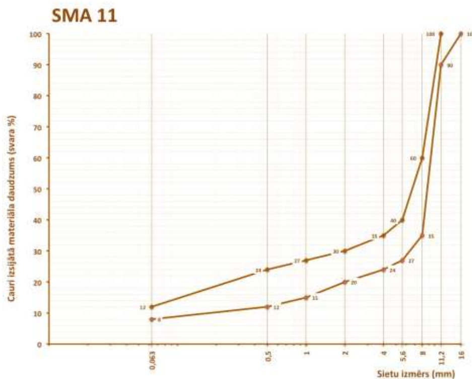
6.2-59 tabula. Prasības šķembu mastikas asfalta SMA 11 granulometriskajam sastāvam
