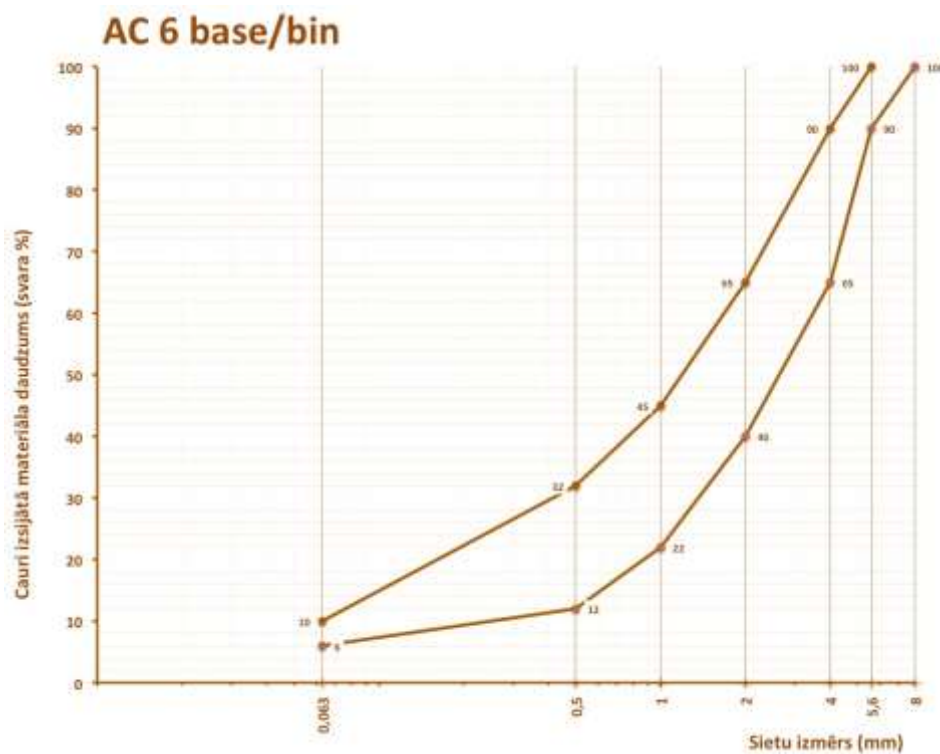
6.2-34 tabula. Prasības karstā asfalta AC 6 base/bin granulometriskajam sastāvam
